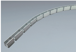
曲線取付用レール (アルミニウム) FN1-EXL-FLEX (1000mm) ¥3,300 器具装着時寸法 ▷
