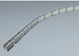
曲線取付用レール (アルミニウム) FN1-EXL-FLEX (1000mm) ¥3,300 器具装着時寸法 ▽
