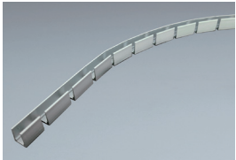
曲線取付用レール (アルミニウム) FN1-EXL-FLEX (1000mm) ¥3,300
