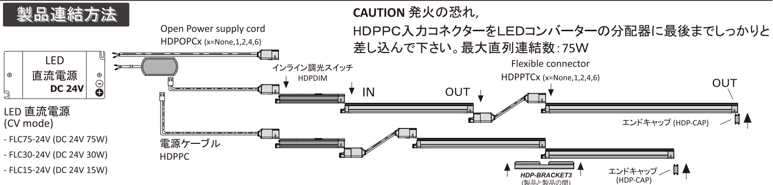
Fig.3 フレックス (HDP2 xxK-24V-C90-FLEX)
