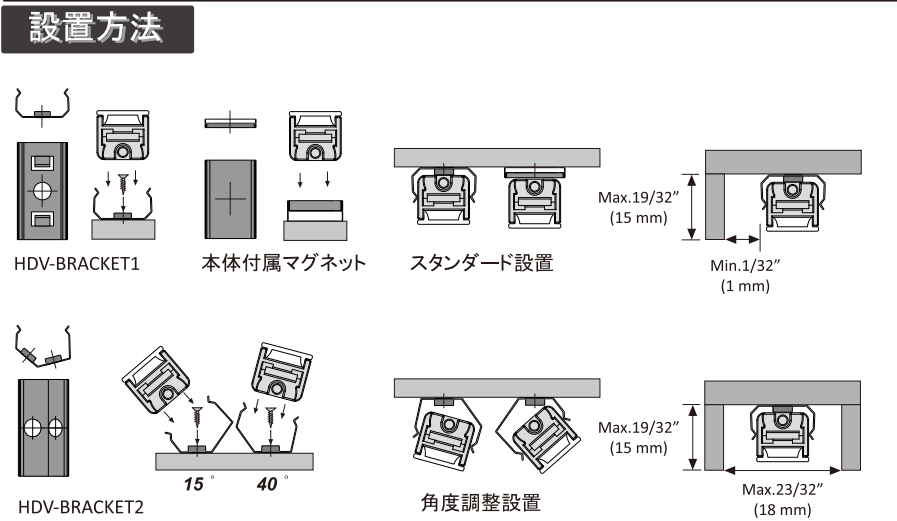
Fig4 Mounting 使用周辺最高温度 : 45℃
