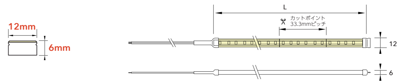
直線取付用レール (樹脂) FTPS-EXLP (1200mm) ¥1,800
