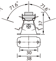
角度調節ブラケット FTT-BRACKET3 (2pcs) ¥2,160 器具装着時寸法▷
