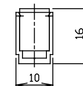
FN1-EXL1取付図
