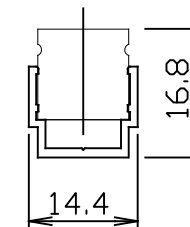
FN2RGB-EXL 取付図
