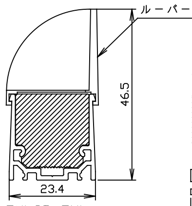
FNL3D-EXL ルーバー 取付図
