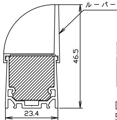
FNL3D-EXL ルーバー 取付図
