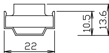
FTT-EXL FT-BRACKET1 取付図
