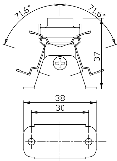
FTT-EXL FT-BRACKET3 取付図
