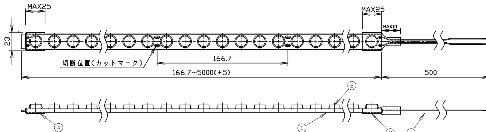
FTT-EXL FT-BRACKET3 取付図
