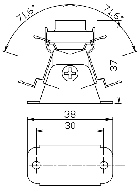
FTT-EXL FT-BRACKET1 取付図
