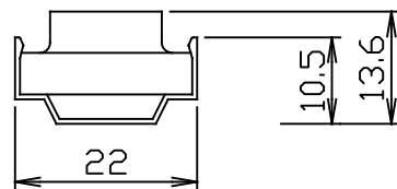
FTT-EXL FT-BRACKET1 取付図
