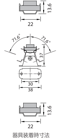
器具装着時寸法
