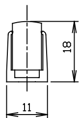
FN1RGB取付図
