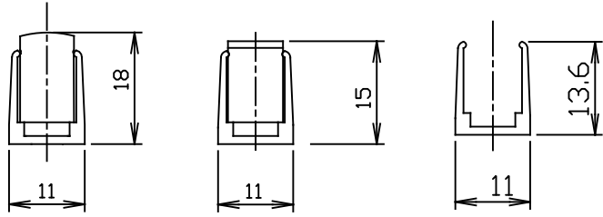
FN1RGB取付図
