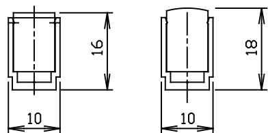
FN1取付図
