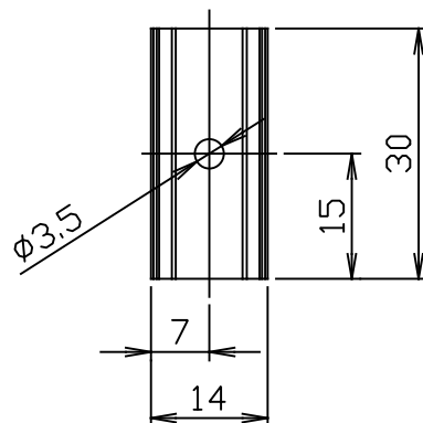
FN2RGB器具取付図
