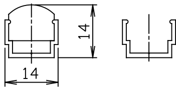
器具取付図
