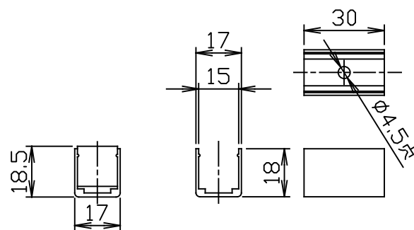
器具取付図
