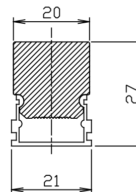
器具取付図
