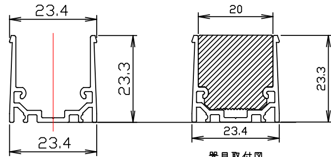
器具取付図
