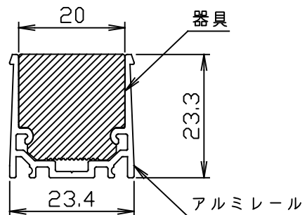
器具取付図
