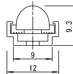
器具取付図
