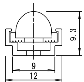
器具取付図
